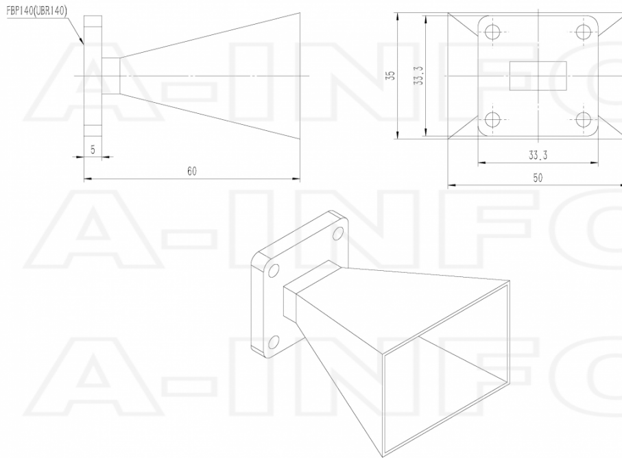
FBP140 Output (P/N: LB-62-15-A)
